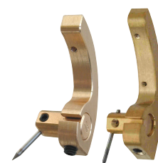
Adaptér elektrody pro OW 38S, OW 76S
